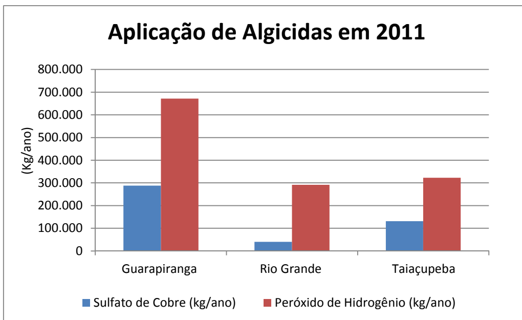
Gráfico 4.10 – Algicidas aplicados nos reservatórios em 2011 (dados fornecidos pela SABESP)
