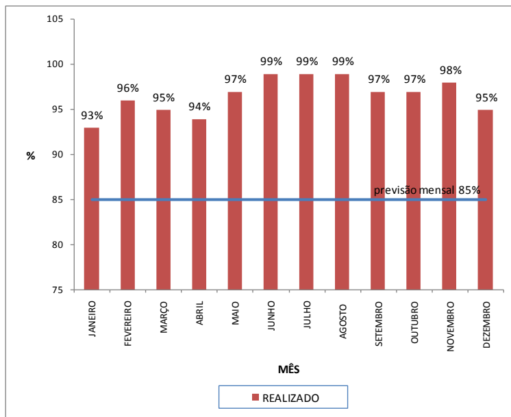
Gráfico 1: Comparativo mensal da razão, em porcentagem, do tempo previsto pelo tempo real de operação das estações de monitoramento do ar durante o ano de 2012.
