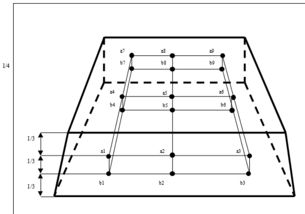
Figura 2 - Seção Longitudinal
